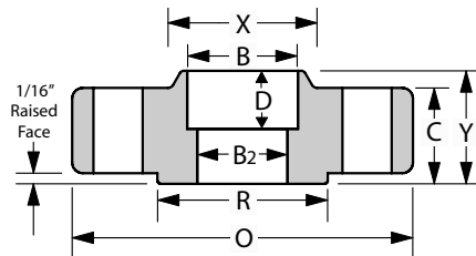
SOCKET WELD (SW)
